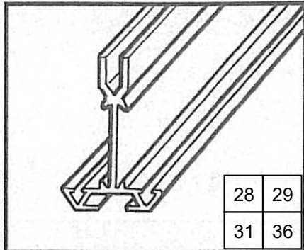
GLAZING BAR
