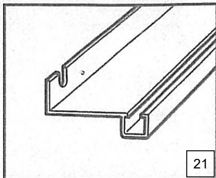
DOOR END CILL
