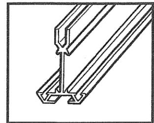
GLAZING BAR
